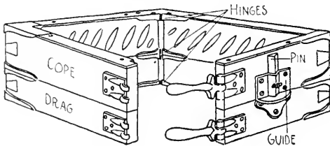
FIG. 496. SNAP FLASK.
